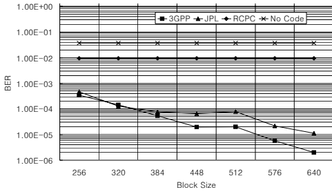
그림 10. 블록크기를 변화시킬 때 오류정정 기법의 BER 성능 비교 (채널 부호화율: 1/2, Eb/No: 2.0dB)
