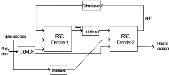
그림 3. Turbo 복호화기
