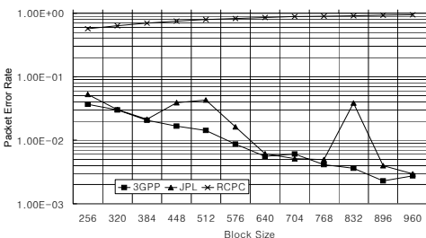
그림 13. 블록크기를 변화시킬 때 오류정정 기법의 packet error rate 성능 비교 (채널 부호화율: 4/7, Eb/No: 2.0dB)
