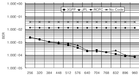
그림 11. 블록크기를 변화시킬 때 오류정정 기법의 BER 성능 비교 (채널 부호화율: 4/7, Eb/No: 2.0dB)
