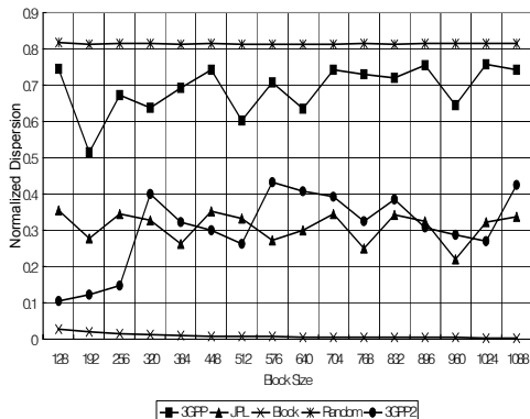
그림 5. 각 인터리버에 대한 정규화된 산포도
