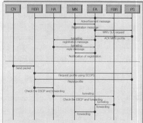
그림 4. 정책 시나리오에 따른 동작 절차 예.
