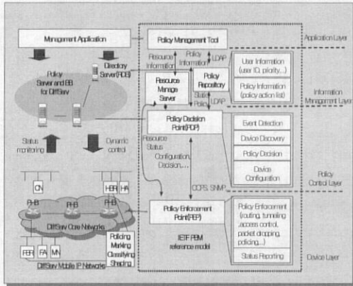
그림 2. 인터넷 QoS 지원 정책기반 이동 IP 망의 프레임워크
