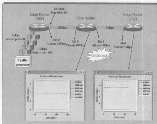
그림 12. 성능 평가 구조 및 대역폭 분석 결과.
