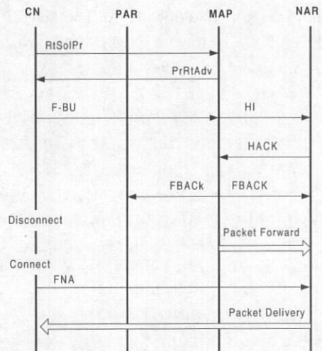
그림 2. F-HMIPv6에서의 등록 및 패킷전달 절차
