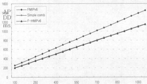
(b) T CM 에 따른 평균 패킷 전달 지연 (T MT =3,000ms, T MA =100ms)
