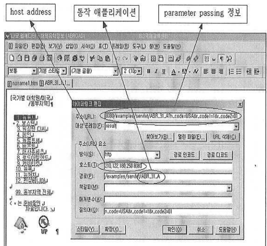
그림 5. 사용자 인터페이스와 응용프로그램의 연동
