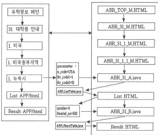
그림 5. 데이터베이스 응용프로그램의 구조 및 동작
