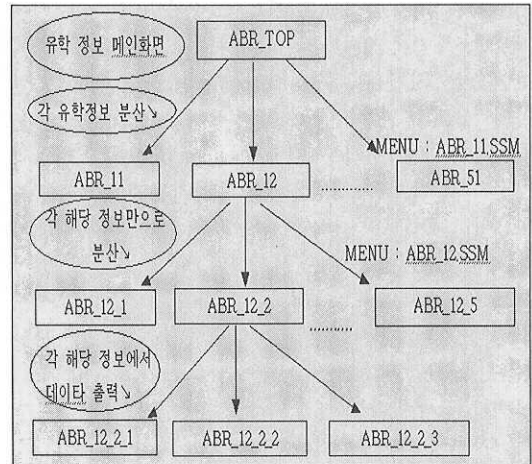
그림 3. 하이퍼텍스트와 GUI에 기반을 둔 사용자 인터페이스의 구조
