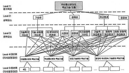
그림 3. Decision Hierarchy
