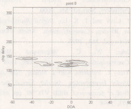
그림 6. 8번 지점에서 신호를 전송하였을 때 수신된 신호를 사용하여 추정된 angle-delay profile
