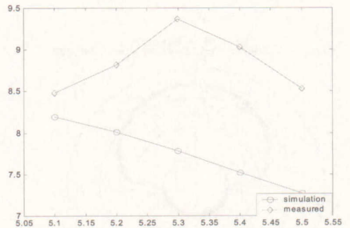
그림 13. 시뮬레이션값과 측정값의 이득 비교 Figure 13. Simulated and measured of gain comparative analysis
