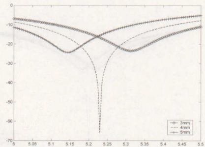
그림 4. L-슬롯 dT 변화에 따른 반사계수 Figure 4. Influence of the dT of L-shaped slot
