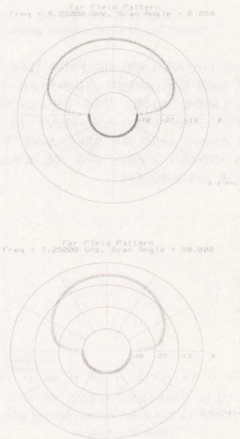
그림 9. 시뮬레이션상의 방사패턴 Figure 9. Simulated E-Plane and H-Plane radiation pattern
