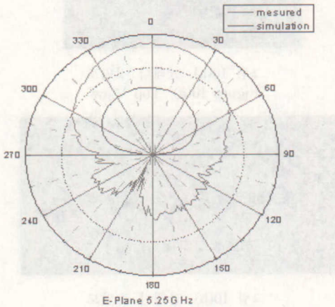
그림 12(a). E-평면 방사패턴 Figure 12(a). E-plane radiation patten
