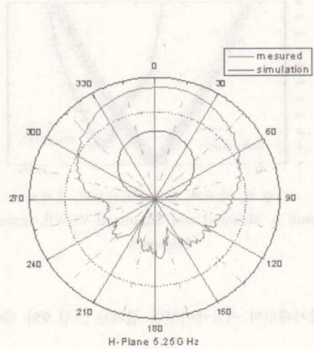
그림 12(b). H-평면 방사패턴 Figure 12(b). H-plane radiation patten
