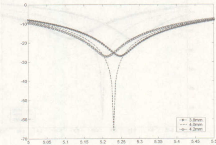
그림 6. 공기층의 두께 t_1 변화에 따른 반사계수 Figure 6. Influence of the thickness of the foam layer on the Return Loss
