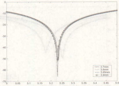
그림 5. 동축 급전의 위치 r_2 변화에 따른 반사계수
