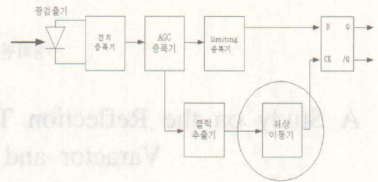
그림 1. Block diagram of optical receiver
