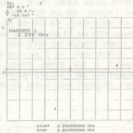
그림 9. Measured phase of -15° at the DC voltage of 0V
