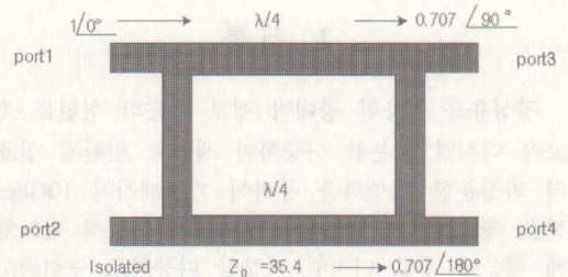
그림 2. Branch Coupler
