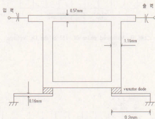
그림 8. Fabricated phase shifter
