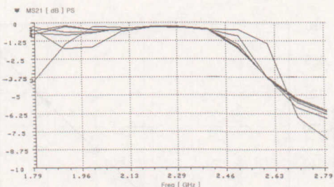
그림 7. Simulation results of insertion loss versus input DC voltage.
