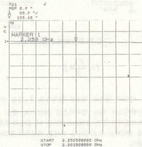
그림 10. Measured phase of 155° at the DC voltage of 12V
