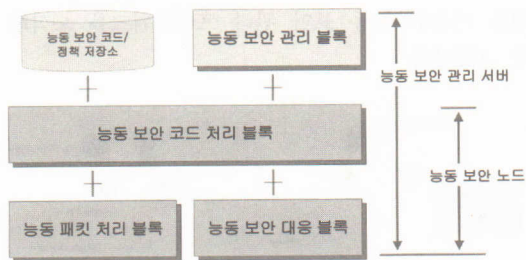
그림 2. 능동 보안 관리 시스템 구성도
