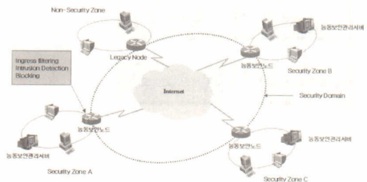
그림 1. 능동 보안 관리 프레임워크
