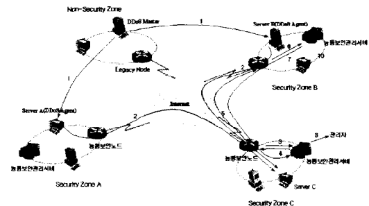
그림 5. DDoS 공격 탐지 및 대응 메커니즘
