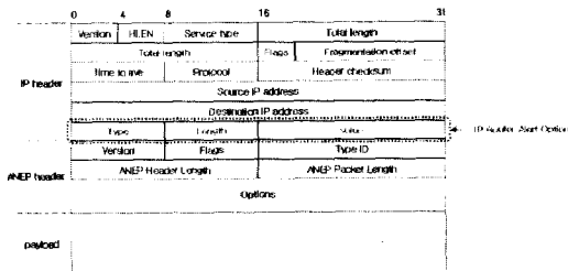
그림 3. 능동 패킷 구조
