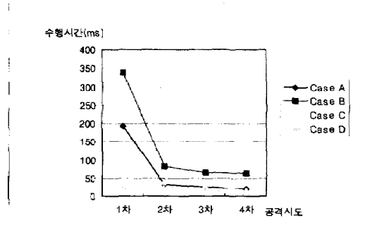
그림 7. 위조 IP 역추적 및 역추적보고 코드 수행시간
