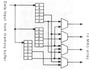
그림 5. 프리-버퍼의 구조
