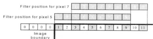
그림 6. DWT 수행시 영상정보의 중복사용 예
