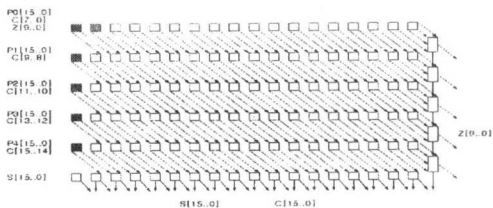
그림 8. MAC에 사용된 CSA 트리
