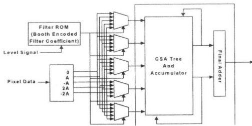
그림 7. MAC의 구조
