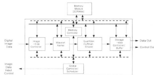
그림 1. 2D DWT 기반 영상압축기의 구조
