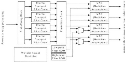
그림 3. 본 논문의 커널 구조
