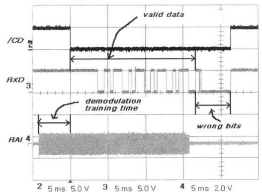
그림 4. RxD, /CD and RAI Signal(Clamped Case)
