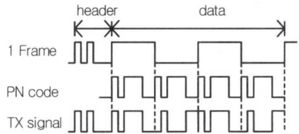
그림 11. Flow Diagram of Digital Data
