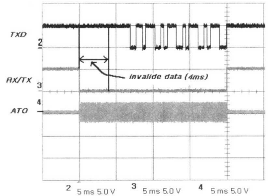
그림 3. TxD, RX/TX and ATO Output Signal
