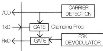
그림 6. Clamping of /CD on RxD
