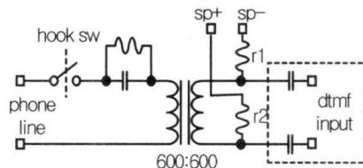
그림 8. Telephone Line Interface
