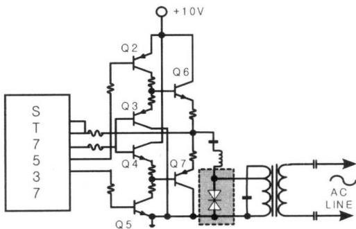
그림 2. Board Schematic
