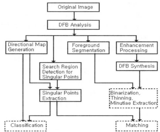
그림 5. DFB의 결과를 이용한 지문영상의 처리과정
