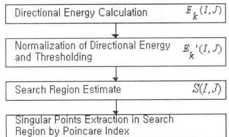
그림 8. 방향성대역영상을 이용한 특이점 추출과정
