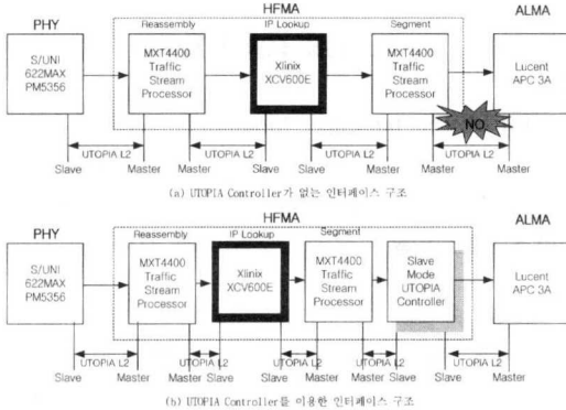
그림 2. MPLS 정합 모듈내의 UTOPIA-L2구조
