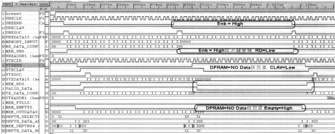
그림 7. DPRAM 상태가 EMPTY일 때 타이밍 시뮬레이션.
