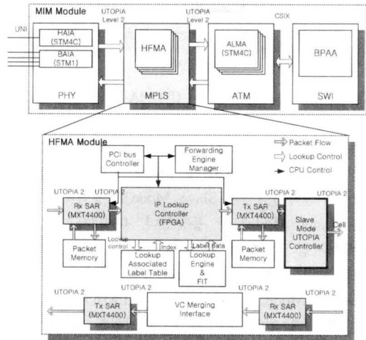
그림 1. MPLS 정합 모듈구조
