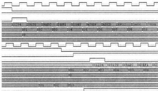
그림 5. Port 0의 타이밍 시뮬레이션 결과.
