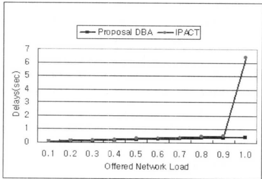
[그림 7] NORMAL 클래스 프레임의 평균지연특성
