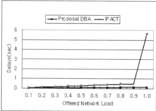
[그림 6] HIGH 클래스 프레임의 평균지연특성
