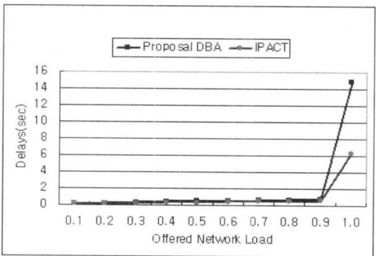
[그림 8] LOW 클래스 프레임의 평균지연특성
