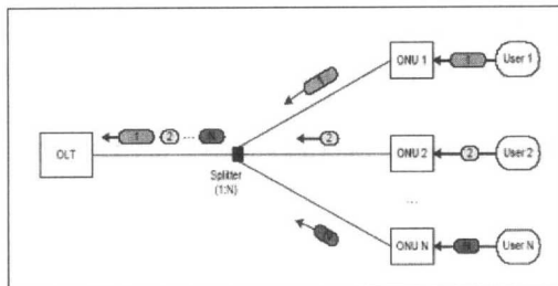
[그림 3] E-PON의 상향(up-stream) 전송 구조[5]
