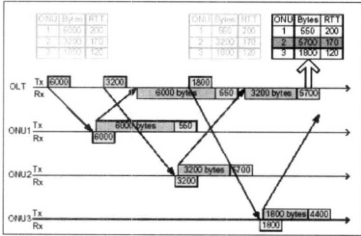
[그림 4] IPACT 대역할당 과정[1]
