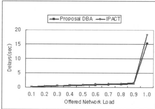
[그림 9] 전체 클래스 프레임의 평균지연특성
