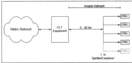
[그림 1] PON 구조
