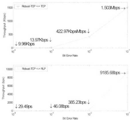
그림 3. 각 알고리즘 간의 Throughput 차이
