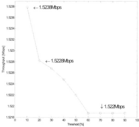
그림 4. 임계값에 따른 Robust TCP의 Throughput 변화
