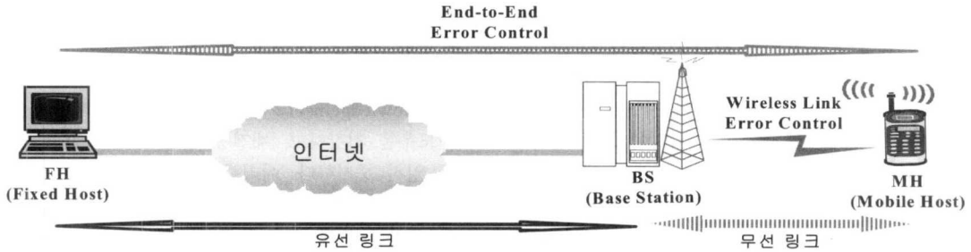
그림 1. FH와 MH의 무선 인터넷 연결 구성도
