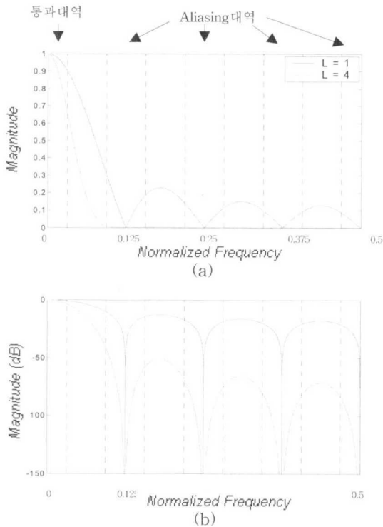
그림 1. CIC 필터의 주파수 응답(M=8, R=1)
