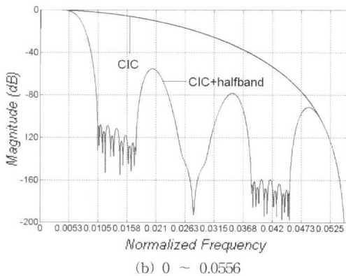
그림 4. 예제 1의 CIC 필터와 half band 필터 등가 주파수 응답
