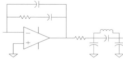
그림 9. 5차 능동형 루프 필터
