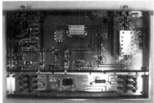
그림 16. DDS Driven PLL 방식 주파수합성기
