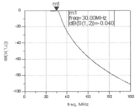
그림 6. DDS 단 LPF 특성
