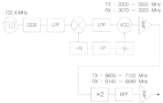
그림 17. 축소된 DDS Driven PLL 방식 주파수 합성기 블록도
