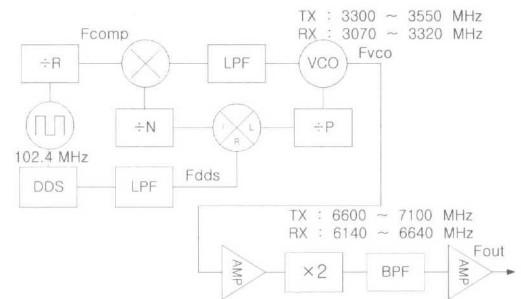
그림 1. PLL with DDS Generated Frequency Offset 방식 주파수합성기 블럭도
