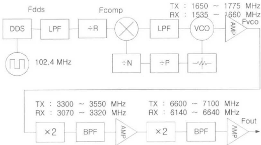
그림 4. DDS Driven PLL 방식 주파수합성기 블럭도
