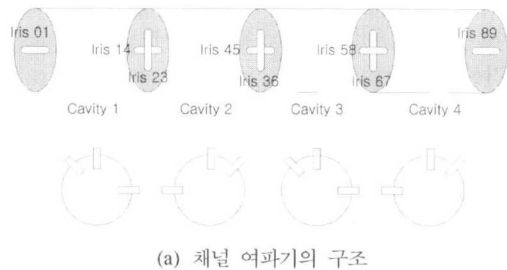
(a) 채널 여파기의 구조
