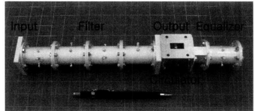
그림 4. 제작한 채널 여파기와 등화기
