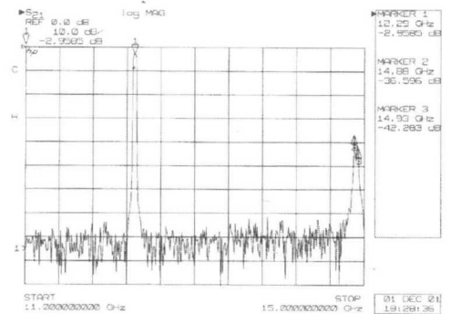
(c) 저지대역 특성 측정 결과
