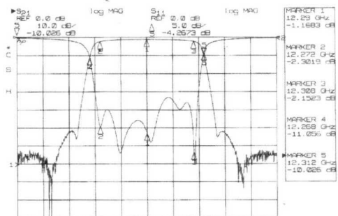
(a) S21 및 S11 측정 결과
