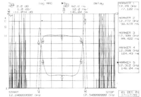
(b) Scaled S21 및 군지연 측정 결과
