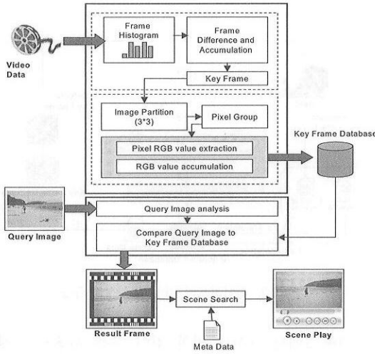
그림 3. 키 프레임 추출 및 특징 검출 구조
