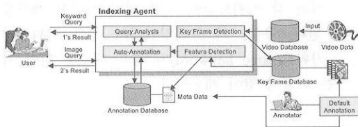
그림 1. 시스템 구조
