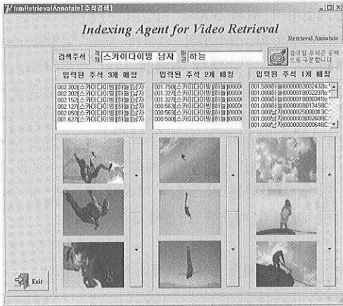
그림 7. 주석기반 검색
