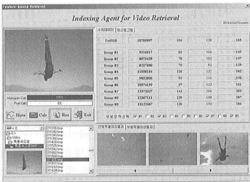
그림 8. 특징기반 검색
