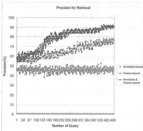
그림 9. 제안 시스템의 검색 정확도
