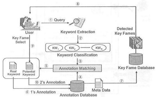
그림 2. 에이전트의 자동 주석처리 구조
