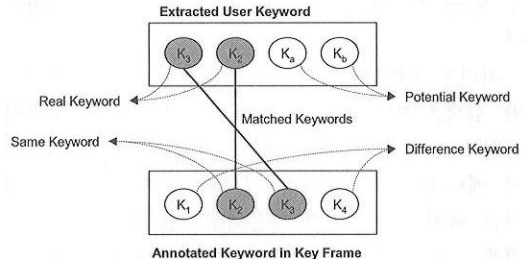
그림 4. 키워드 분류
