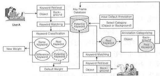
그림 6. 주석 카테고리이징
