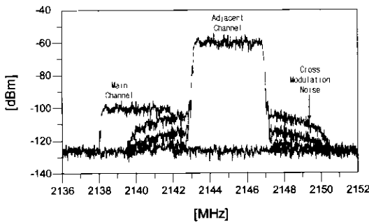
그림 8. LNA 출력에서 Cross-Modulation 잡음
