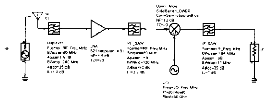
그림 5 W-CDMA 단말기 수신부 블록 회로도
