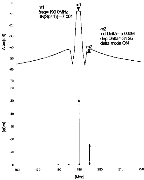
그림 7 인접채널 선택도에 대한 시뮬레이션 결과
