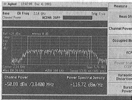
그림 11. IF(190MHz) 출력 파형
