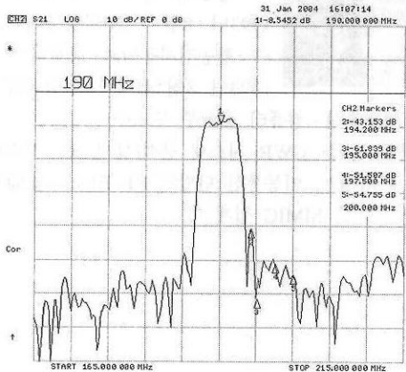
그림 12. IF 채널필터의 ACS 감쇄특성
