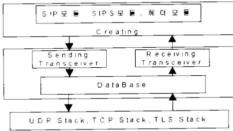
그림 6. sipstack의 구조
