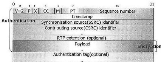
그림 4. SRTP 패킷 형태
