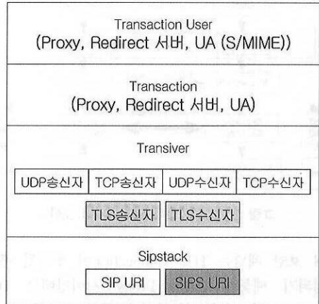
그림 5. 구현된 SIP 프로토콜의 구조
