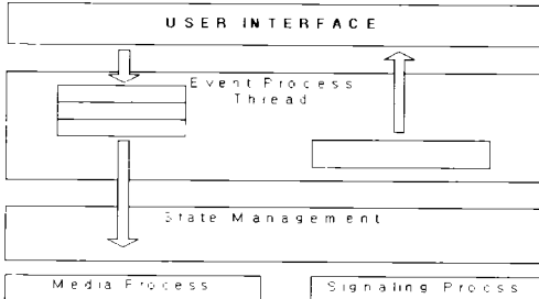
그림 10. 단말기의 설계 및 구조
