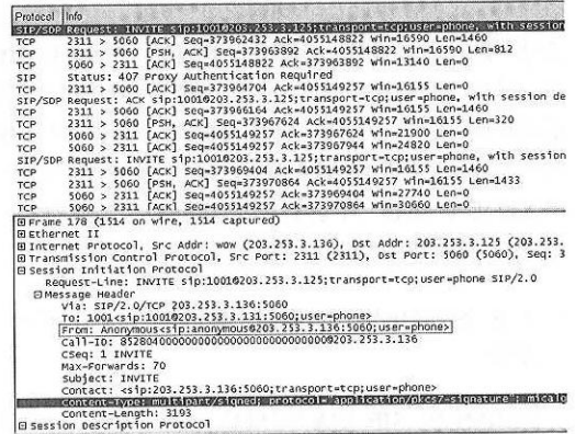
그림 13. SIP 메시지 암호 및 서명 모드가 적용된 SIP 메시지
