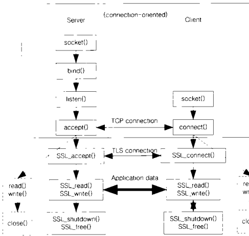
그림 2. TLS를 통한 SIP 메시지 보안
