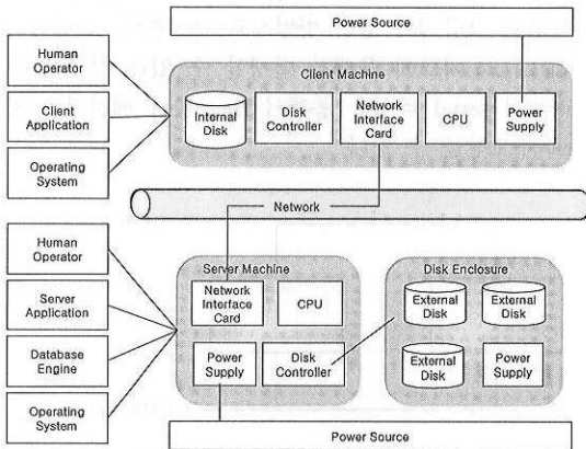
그림 5. SPOF 요소들
