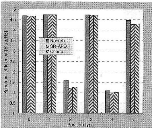
그림 13. Ka-band 도심 환경에서 주파수 효율 비교
