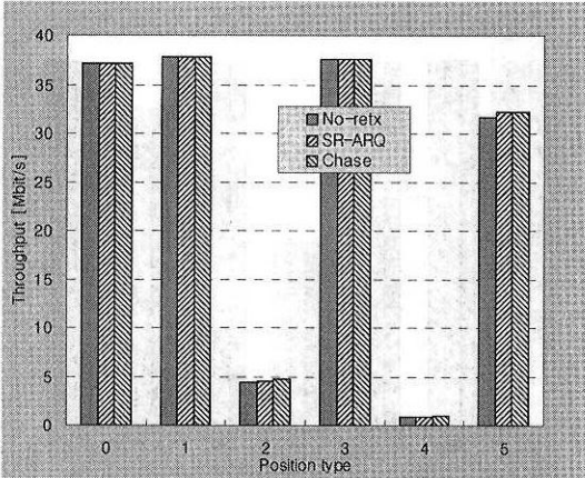
그림 12. Ka-band 도심 환경에서 처리율 비교
