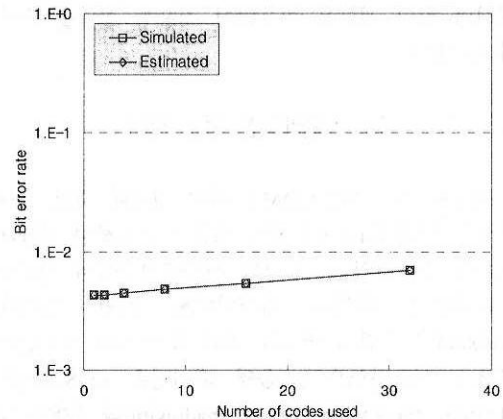
그림 6. 동시 사용 코드 수에 따른 수신 SINR 추정에 의한 BER과 링크 시뮬레이션에 의한 BER 비교 (QPSK, Es/No=15dB).
