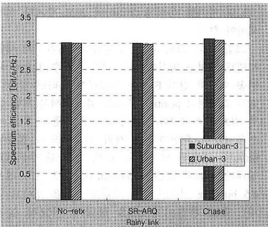
그림 14. 강우 감쇄가 있는 환경에서 주파수 효율 비교
