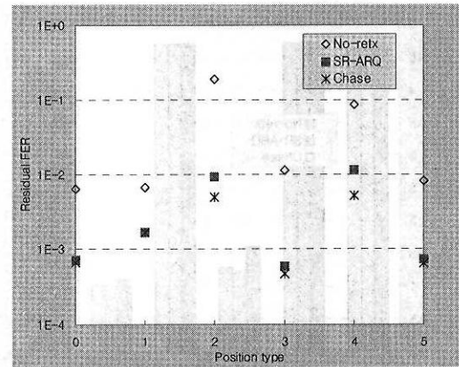
그림 11. Ka-band 도의 환경에서 잔여 FER 비교
