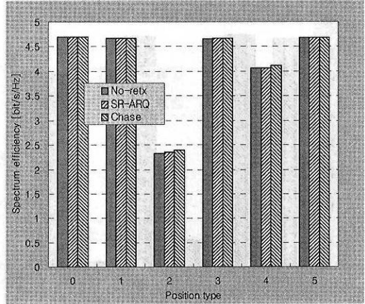
그림 10. Ka-band 도의 환경에서 주파수 효율 비교
