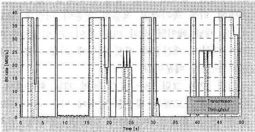
그림 8. 시간 진행에 따른 전송률과 처리율 변화 (Suburban-3).
