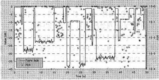
그림 7. 시간 진행에 따른 페이딩과 프레임 오류 변화 (Suburban-3).
