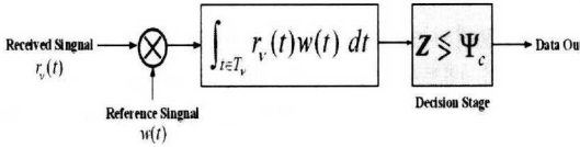
그림 2 : 기존의 Coherent OOK UWB 시스템의 수신기 구조
