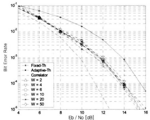
그림 9 : AWGN 채널에서 Noise Power Windowing 슬롯수 W 에 따른 Noncoherent OOK UWB 시스템의 BER 성능 ( C = 20, U = 0.05 ).
