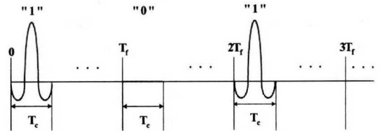
그림 1 : 일반적인 OOK UWB 시스템의 전송 신호 예시.
