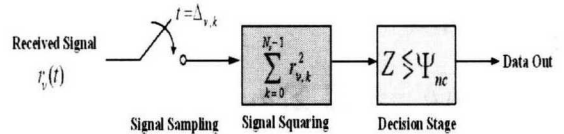
그림 4 : 전력검출 기반의 Noncoherent OOK UWB 시스템 수신기의 일반적인 구조
