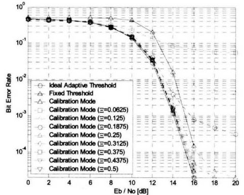
그림 14 : IEEE 802.15 TG3a CM1 실내 무선 채널에서 다중경로에 의한 펄스간 간섭이 존재할 때 Noise Power Calibration 모드가 적용된 Noncoherent OOK UWB 시스템의 정규화된 프레임 시간 T 에 따른 BER 성능 ( N_s = 20 , C = 20 ).
