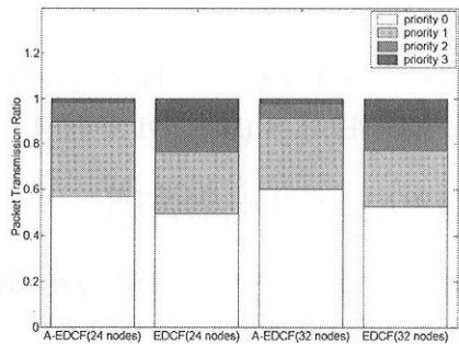
그림 8. 패킷 전송 비율로 나타낸 적응형 EDCF와 EDCF의 우선순위 보장 비교(노드의 수가 24개, 32개인 경우)
