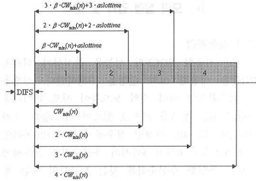
그림 5. 적응형 EDCF의 AIFS의 결정
