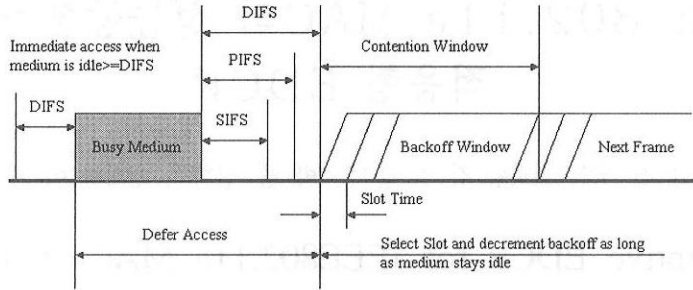
그림 1. 경쟁 구간에서 DCF와 프레임들간 시간 간격(inter-frame space)
