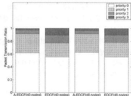
그림 9. 패킷 전송 비율로 나타낸 적응형 EDCF와 EDCF의 우선순위 보장 비교(노드의 수가 40개, 48개인 경우)
