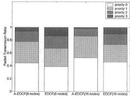
그림 7. 패킷 전송 비율로 나타낸 적응형 EDCF와 EDCF의 우선순위 보장 비교(노드의 수가 8개, 16개인 경우)
