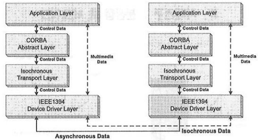
그림 4. 등시성 데이터의 실시간 송수신 구조
