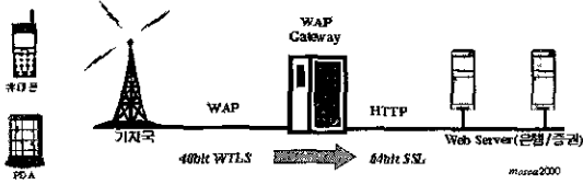
그림 2 3 WAP에서 WTLS-SSL 프로토콜
