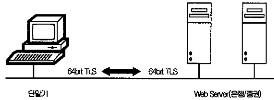
그림 2 1 유선환경에서의 TLS프로토콜
