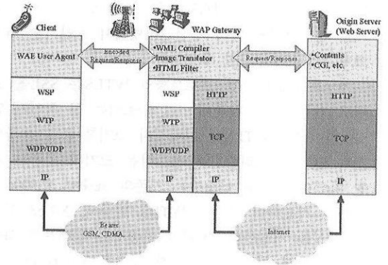
그림 2.7. WTLS-SSL프로토콜 변환
