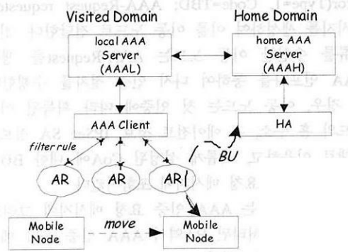
그림 6. 동일 AAA 클라이언트 내 핸드오프 처리
