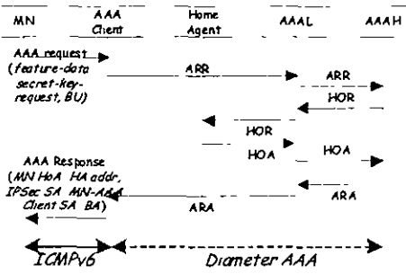
그림 5 확장된 AAA Model의 정보 흐름도
