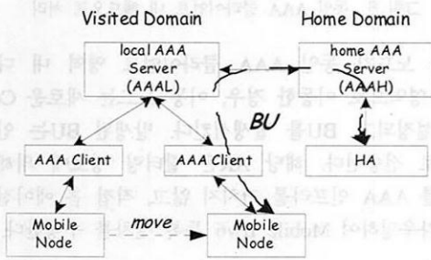
그림 8. 다른 AAA 클라이언트 간 핸드오프 처리
