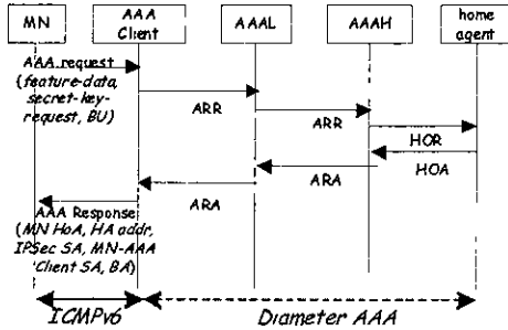
그림 3 기본 AAA Model의 정보 흐름도
