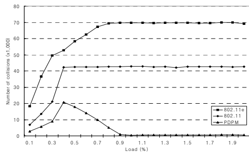
그림 10. 부하의 증가에 따른 충돌 횟수의 비교
