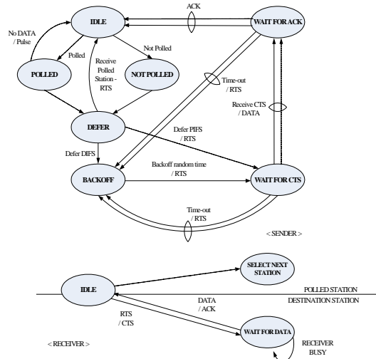
그림 8. PDPM 프로토콜의 상태 천이도
