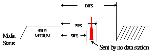
그림 6. 선택된 스테이션에 의한 펄스의 사용
