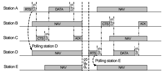
그림 7. 우선순위 기반 분산 폴링 매커니즘(PDPM)의 묘사.
