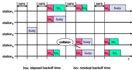
그림 1. DCF 모드에서의 백오프 매커니즘
