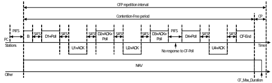
그림 2. PCF 모드에서의 폴링 매커니즘
