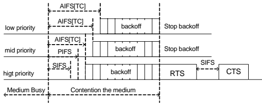
그림 3. EDCA 모드에서의 매체 접속 순위
