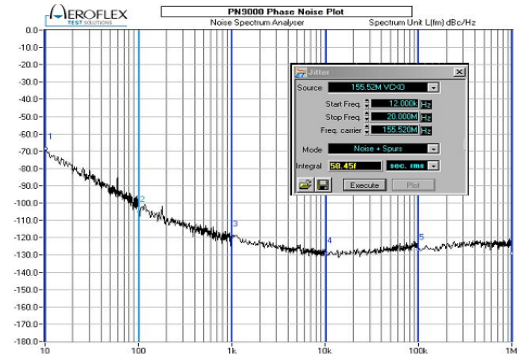
그림 8. 위상잡음 특성
