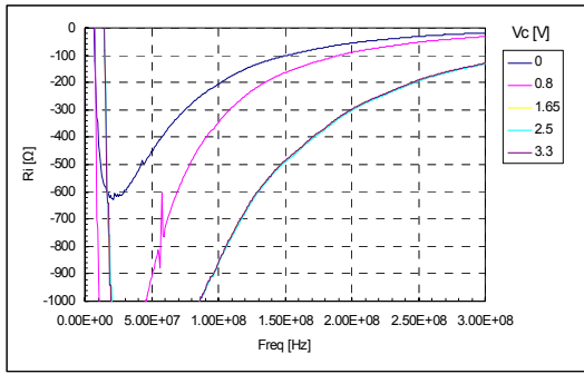
(a) 부성저항 특성
