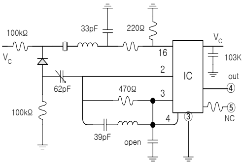
(b) 회로도
