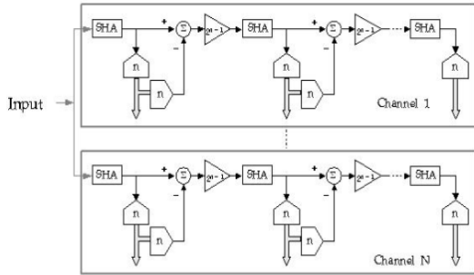
그림 2. 병렬 파이프라인 A/D 변환기의 블록도
