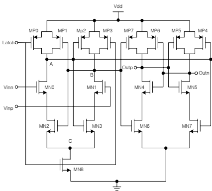
그림 8. 비교기 회로
