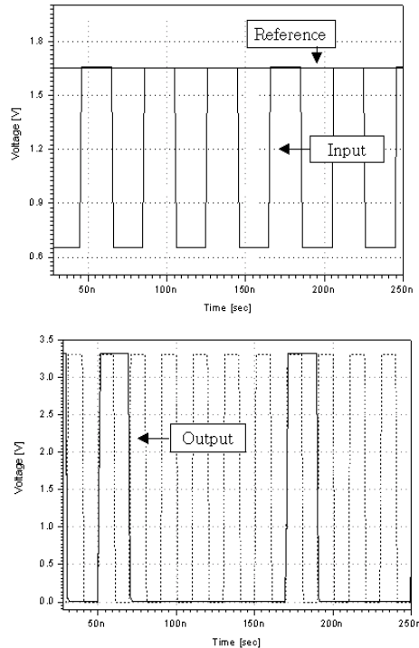
그림 9. 비교기의 Overdrive recovery 시뮬레이션 결과
