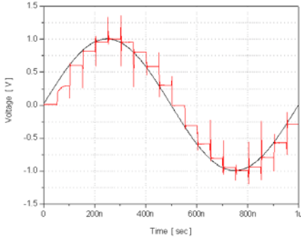
그림 7. SHA 셀의 출력파형
