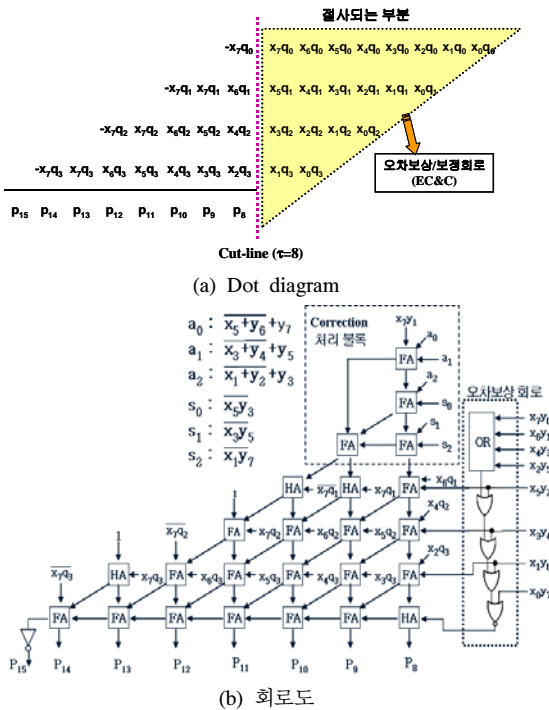
그림 4. 오차보상을 갖는 8-비트x8-비트 Booth 승산기( \tau=8 인 경우)
