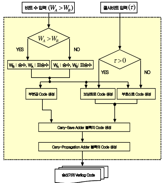
그림 5. VPM_Gen의 흐름도
