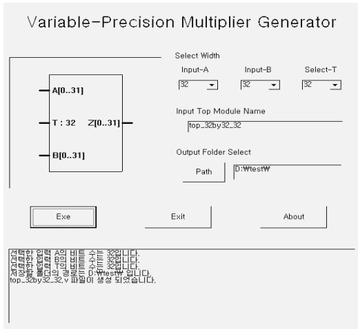
그림 6. VPM_Gen의 실행화면
