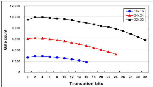
그림 10. \tau 에 따른 승산기의 게이트 복잡도
