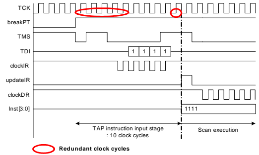
그림 5. 기존의 TAP 컨트롤러의 제어 타이밍도
