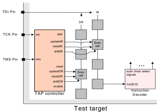
그림 4. 기존의 TAP 컨트롤러의 출력신호
