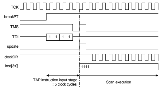
그림 8. 개선된 TAP 컨트롤러의 제어 타이밍도
