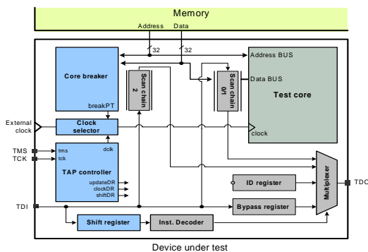
그림 10. 데모시스템 : 디버깅 유닛을 탑재한 테스트 코어
