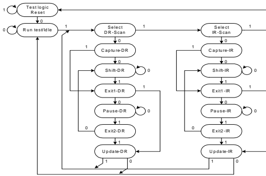
그림 3. 기존의 TAP 컨트롤러 상태모 5)
