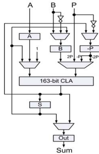
그림 3. 모듈러 덧셈 곱셈기 구조
