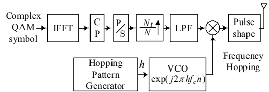
그림 2. FH-OFDMA 송신기
