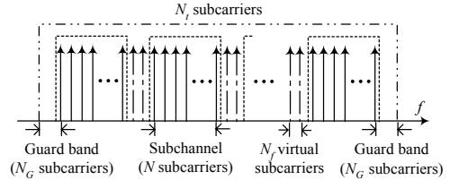
그림 1. 다중사용자 FH-OFDMA의 부반송파 배치
