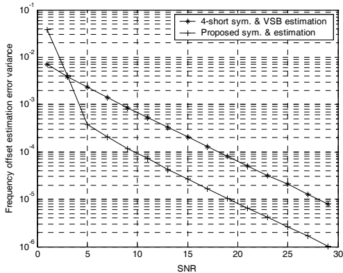
그림 9. 주파수 오프셋 추정 오차 비교 (AWGN 채널, \Delta = 0.25 )
