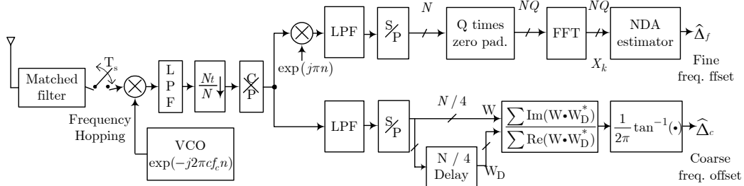
그림 5. 제안한 대략적 주파수 오프셋 추정 및 미세 주파수 오프셋 추정 알고리즘 블록도 그림
