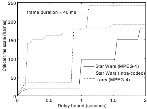
그림 2. 허용 지연 d 의 변화에 따른 임계 시간 준위( t_c ) 변화
