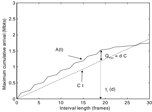
그림 1. 임계 시간 준위( t_c )의 정의
