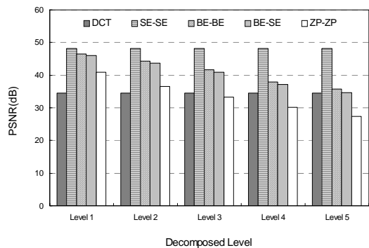
그림 9. 고정소수점 검증을 통한 경계처리 방식들의 PSNR 결과
