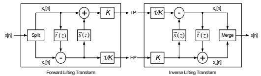
그림 1. 팩토링을 이용한 정방향역방향 리프팅 방식의 구조도 Fig 1. Forward/inverse lifting scheme using factoring
