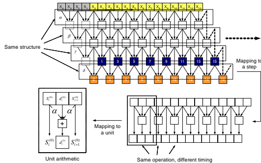
그림 4. 1차원 리프팅의 구조사상을 통한 단위연산
