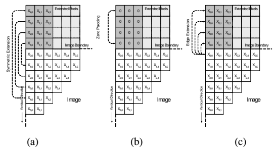
그림 8. 제한한 경계처리 방식 (a) 대칭적 확장 (b) 영값 확장 (c) 가장자리 확장
