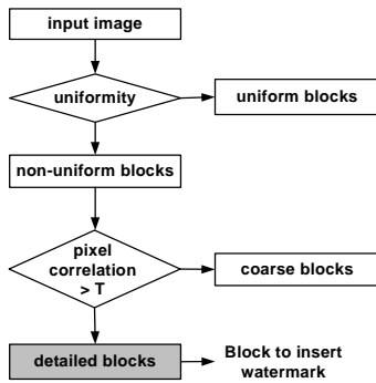
그림 2. 워터마크 삽입 블록의 선정과정 Fig 2. Procedure to select the blocks to insert watermark in
