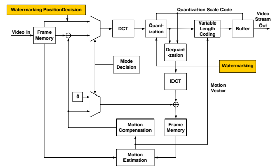
그림 1. MPEG-2 엔코더와 워터마킹 위치 Fig 1. MPEG-2 encoder and watermarking position
