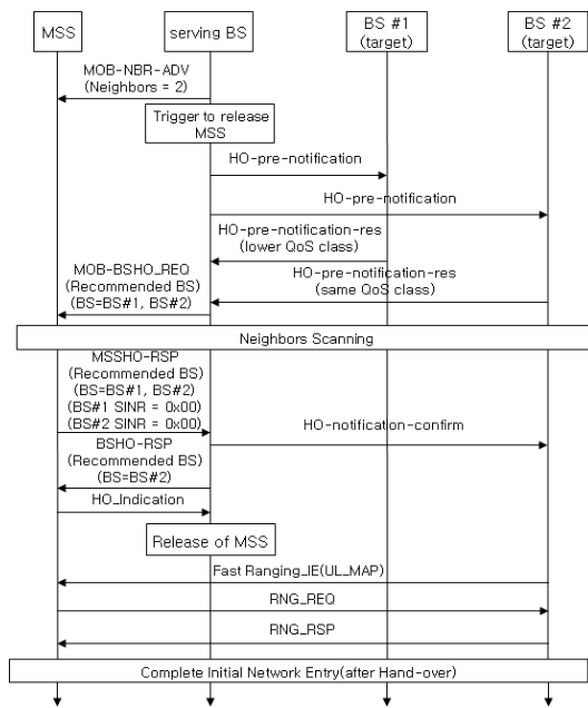
그림 2. BS 요청에 의한 핸드오버 처리
