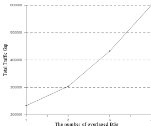
그림 12. BS의 위치에 따른 트래픽량
