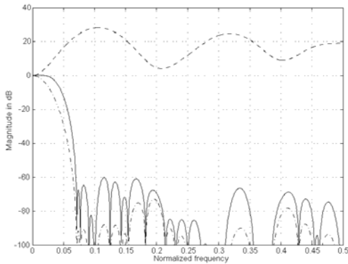
그림 3. 예제 1의 CP 전처리기 주파수 응답 (일점쇄선), ISOP 등화기 응답 (끊어진 선), 전체 응답 (실선)
