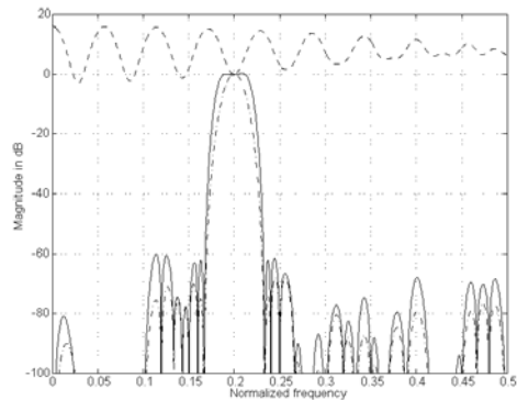
그림 1. 전처리-등화기 구조의 대역 통과 여파기 주파수 응답: 전처리 (일점쇄선), 등화기 (끊어진 선), 전체 여파기 (실선)
