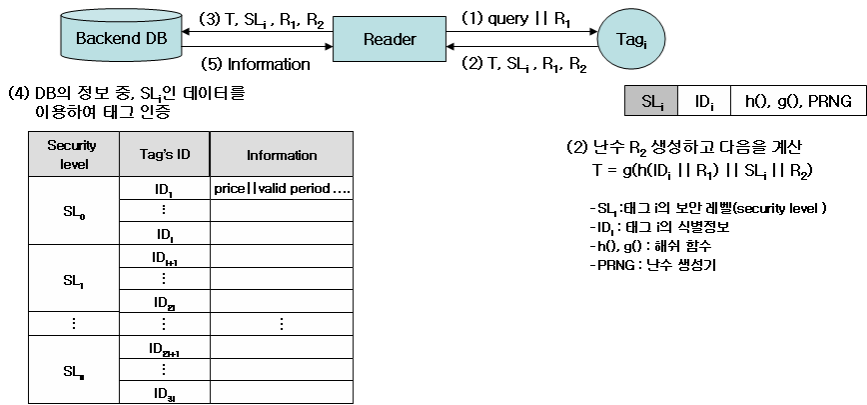
그림 8. Security level based Randomized authentication protocol
