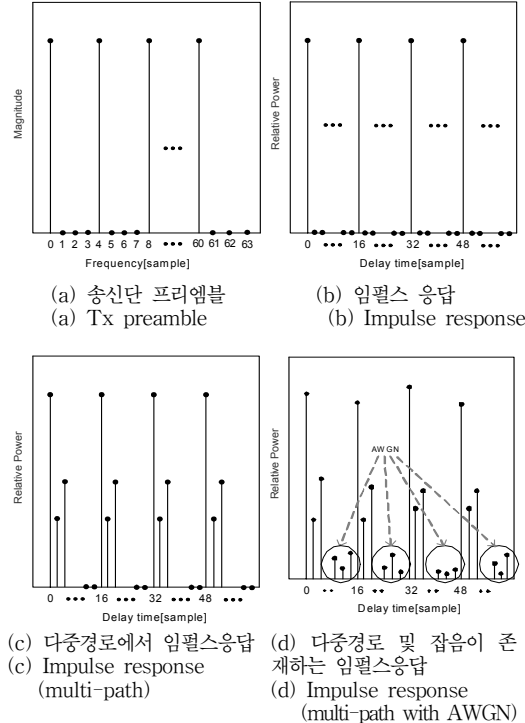
그림 3. 송신단의 프리엠블과 임펄스 응답의 예 Fig. 3. Tx preamble and Impulse response examples
