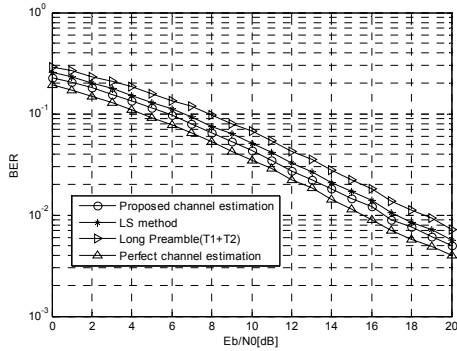
그림 12. 실외환경에서 4개의 다중경로를 가질 때 BER 곡선전폭 감쇄 0.7 Fig. 12. BER curves in 4 path outdoor environment
