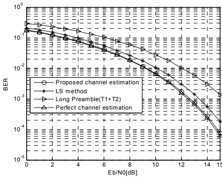
그림 9. 실내환경에서 4개의 다중경로를 가질 때 BER 곡선 Fig. 9. BER curves in 4 path indoor environment
