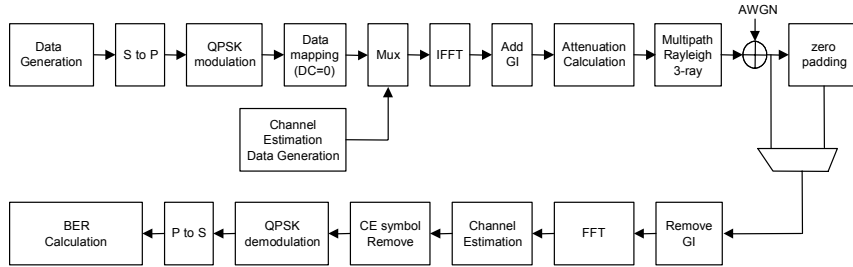
그림 5. 시뮬레이션 모델링 블록도 Fig. 5. Simulation model block
