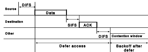
그림 3. 802.11a CSMA/CA 기반 DCF프로토콜의 동작
