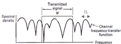
그림 3. Typical frequency-selective and flat fading ( B_c < W )
