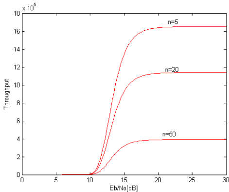
그림 12. 단말수에 따른 E_b/N vs. throughput
