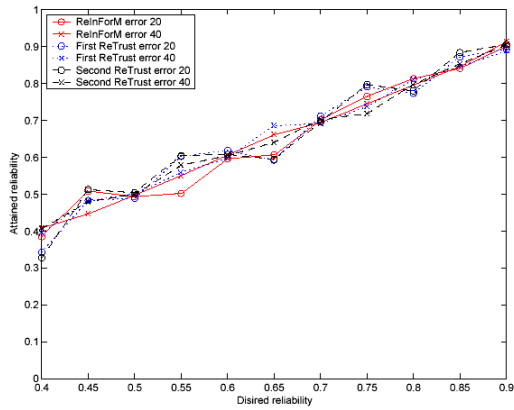
그림 10. 소스 노드의 신뢰도와 sink 노드의 신뢰도 비교 Fig. 10. Attained reliability vs. desired reliability
