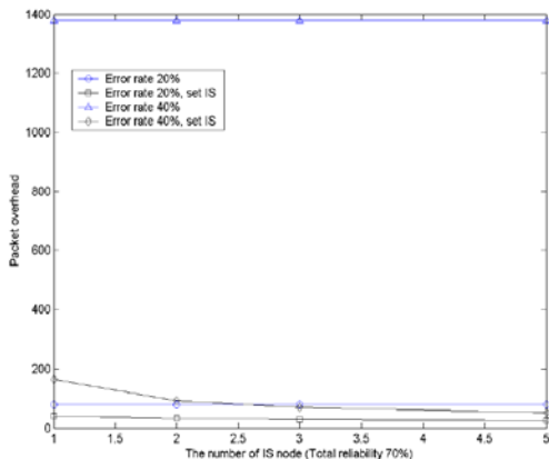
그림 8. Multi-IS 노드 설정시 총 패킷 오버헤드. Fig. 8. Total packet overhead with multi-IS node.
