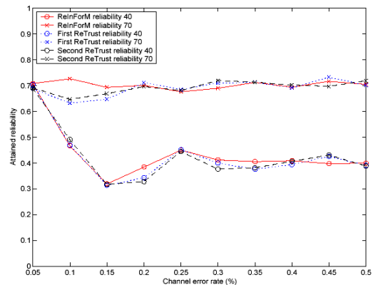
그림 9. 채널 에러율 증가에 따른 sink 노드의 신뢰도 비교. Fig. 9. Attained reliability under increasing channel error rate
