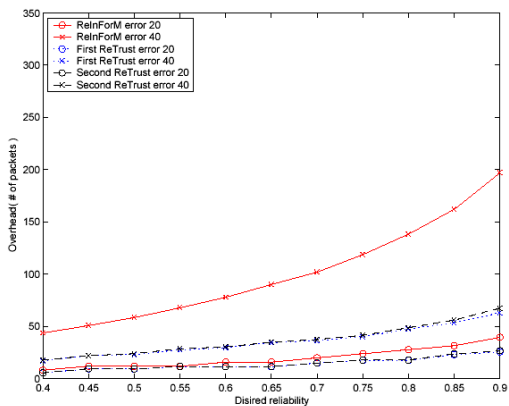
그림 12. 요구 신뢰도 변경에 따른 패킷 오버헤드 비교 Fig. 12. Packet overhead for varying desired reliability
