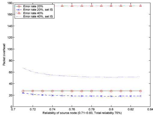
그림 7. 소스 노드의 전송 신뢰도를 변경하였을 때 총 패킷 오버헤드 비교( 신뢰도 70% 일때). Fig. 7. Total packet overhead for varying reliability between the source and the IS (total reliability of 70%).
