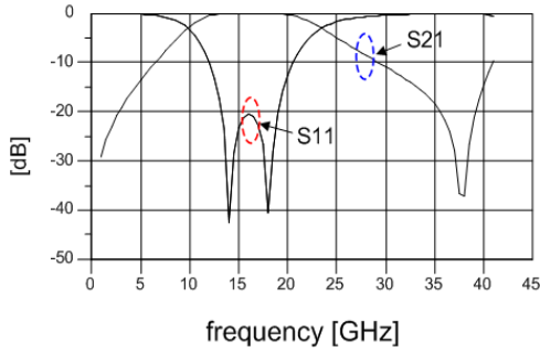
그림 3-2. 제안된 Sub-harmonic 혼합기의 LO 정합특성
