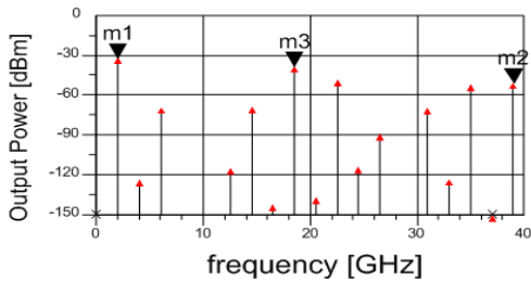
그림 3-3. 제안된 Sub-harmonic 혼합기의 출력 스펙트럼
