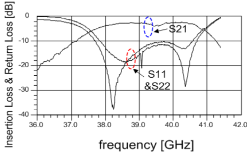
그림 4-3. 대역통과 여파기의 측정결과
