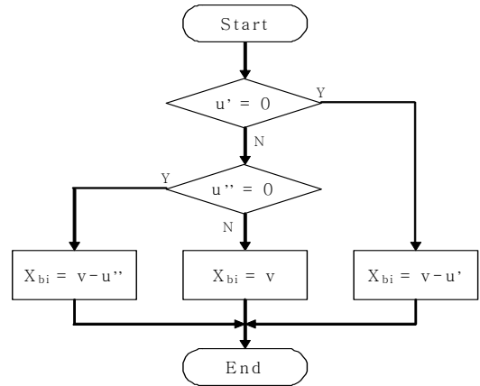
그림 9. 간섭제거 알고리즘
