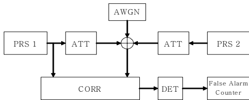
그림 11. 시뮬레이션 모델
