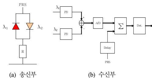
그림 3. 송·수신부의 구조
