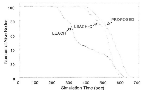
그림 6. 센서망 생존시간 성능
