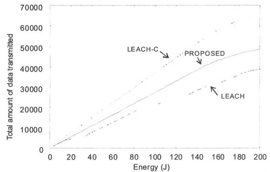
그림 9. 소요 에너지에 따른 데이터 전송량
