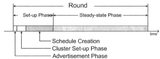
그림 1. LEACH의 한 라운드에서의 동작 과정
