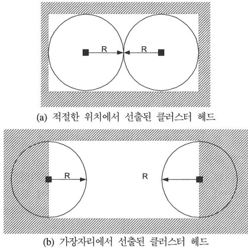
그림 5. 반경 R 과 클러스터 헤드의 브로드캐스트 범위 ( k=2 인 경우)
