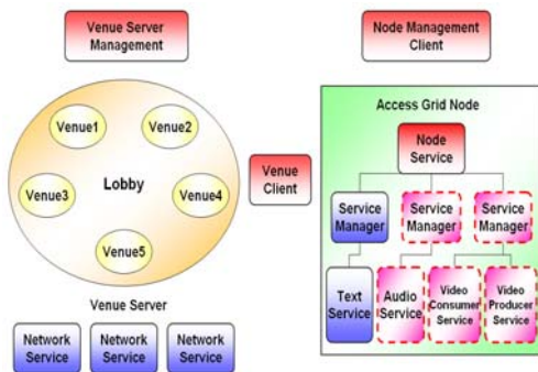
그림 1. AGTk의 구조
