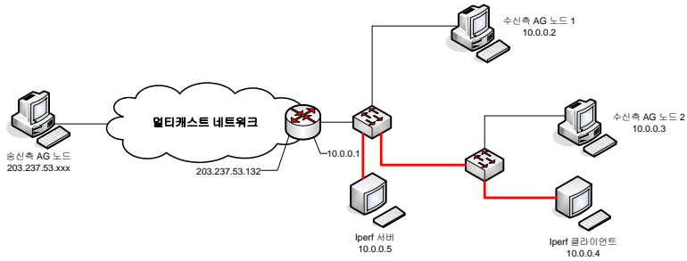
그림 9. 테스트 베드
