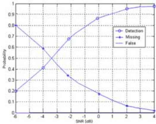
그림 13. 제안된 시간동기화 알고리즘 성능 Fig. 13. Performance of the proposed timing synchronization algorithm
