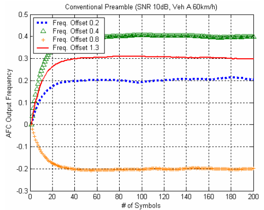
그림 12. AFC의 주파수 오프셋 추정 성능 (10dB SNR). Fig. 12. AFC Performance of Frequency Offset Estimation (10dB SNR)
