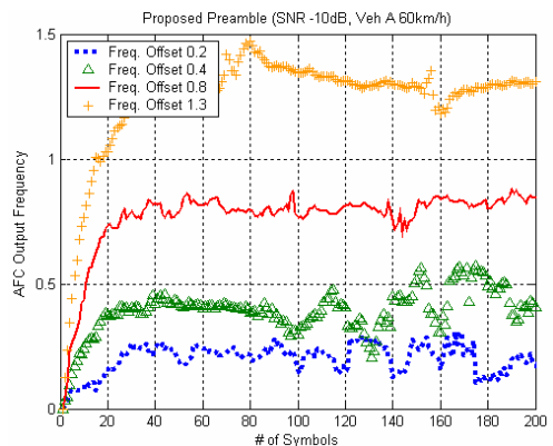
그림 16. AFC의 주파수 오프셋 추정 성능 (-10dB SNR) Fig. 16. AFC Performance of Frequency Offset Estimation (-10dB SNR)
