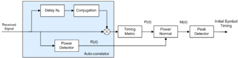
그림 2. 초기 심볼 타이밍 동기화 블록 다이어그램 Fig. 2. Initial timing synchronization block diagram
