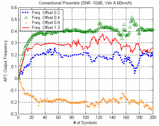
그림 11. AFC의 주파수 오프셋 추정 성능 (-10dB SNR). Fig. 11. AFC Performance of Frequency Offset Estimation (-10dB SNR)
