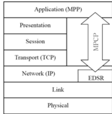
그림 2. MPP 프로토콜 구조
