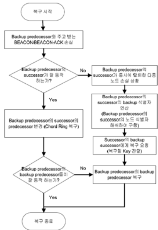
그림 9. 다중 노드 손실 복구를 위한 backup successor 동작 과정
